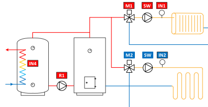
8. Circuit 2 et eau chaude sanitaire vanne fermée
